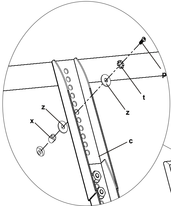
M4 Diameter Bolt
